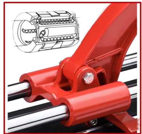
Coulisseau sur roulements à billes linéaires
